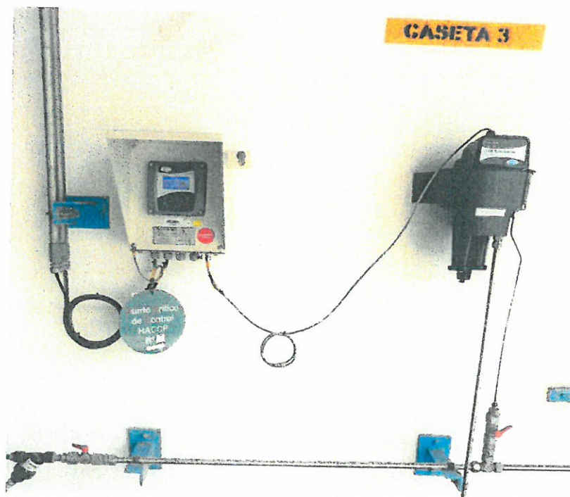
INDICADOR- TRANSMISOR Y SENSORES DE TURBIDEZ AE-30-006
