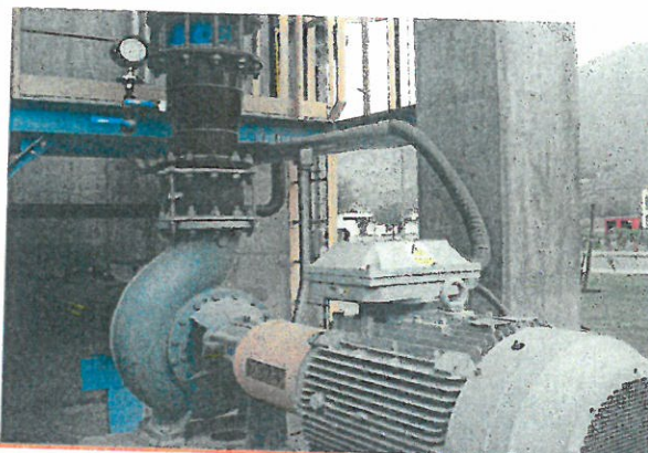
CONJUNTO MOTOR-BOMBA BC-30-02A
