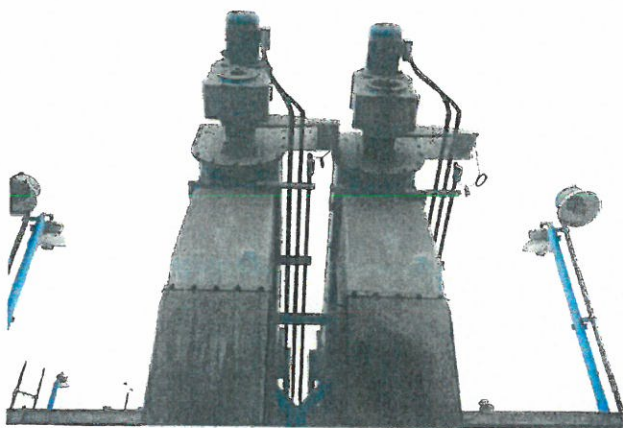
ROSCAS ETRACTORAS DE ARENA
