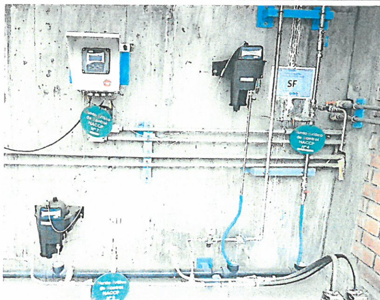
INDICADOR- TRANSMISOR Y SENSORES DE TURBIDEZ AE-30-002/007
