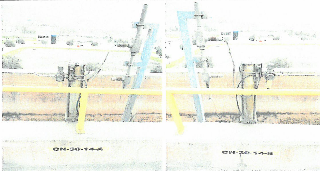
COMPUERTAS NEUMATICAS ENTRADA A FILTROS CN-30-14 A/B
