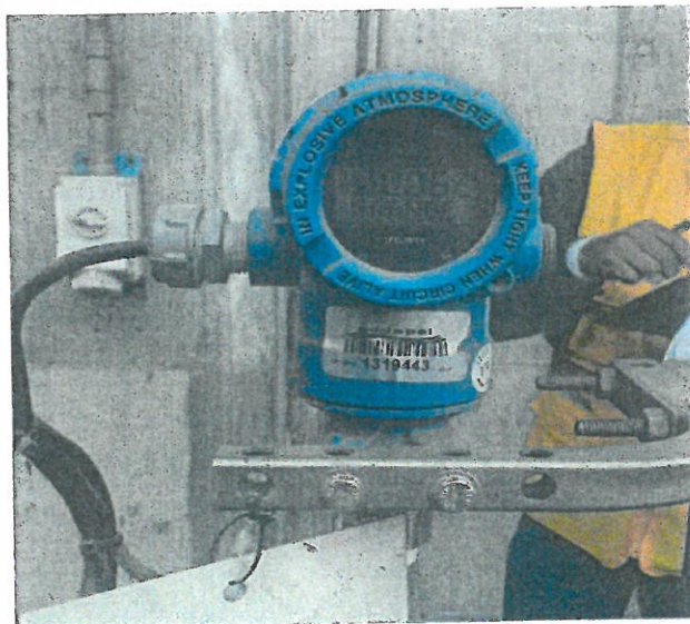
SENSOR E INDICADOR-TRANSMISOR DE PRESION PIT-30-002
