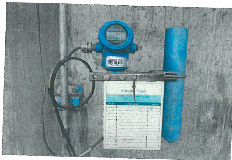
SENSOR E INDICADOR-TRANSMISOR DE PRESION PIT-20-001
