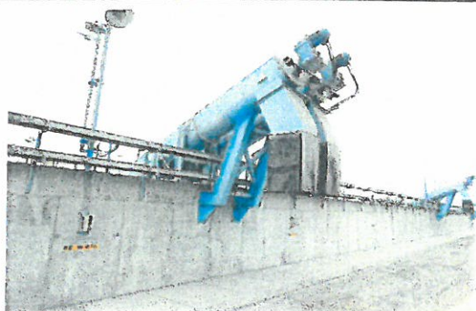
ROSCAS ETRACTORAS DE ARENA
