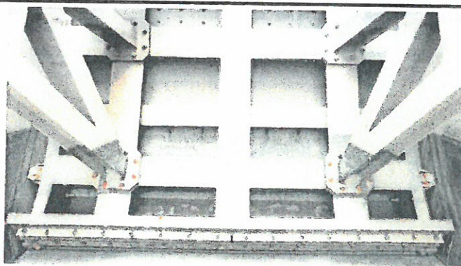
COMPUERTA RADIAL, PRESENCIA DE OXIDO
