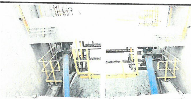
CILINDROS HIDRAULICOS COMPUERTA
