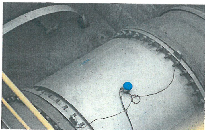
SENSOR E INDICADOR-TRANSMISOR DE CAUDAL FE/FIT-10-001B
