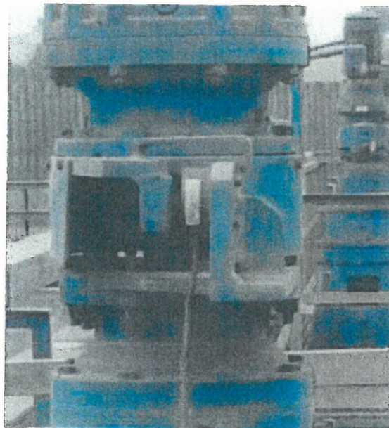
SENSOR E INDICADOR-TRANSMISOR DE TORQUE WE/WIT 10-001H
