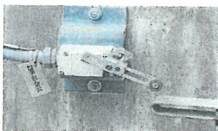
SENSOR LIMITE DE CARRERA
