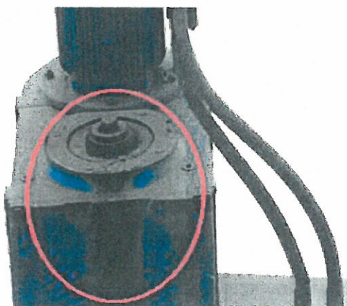
PRESENCIA DE OXIDO Y FUGA DE ACEITE
