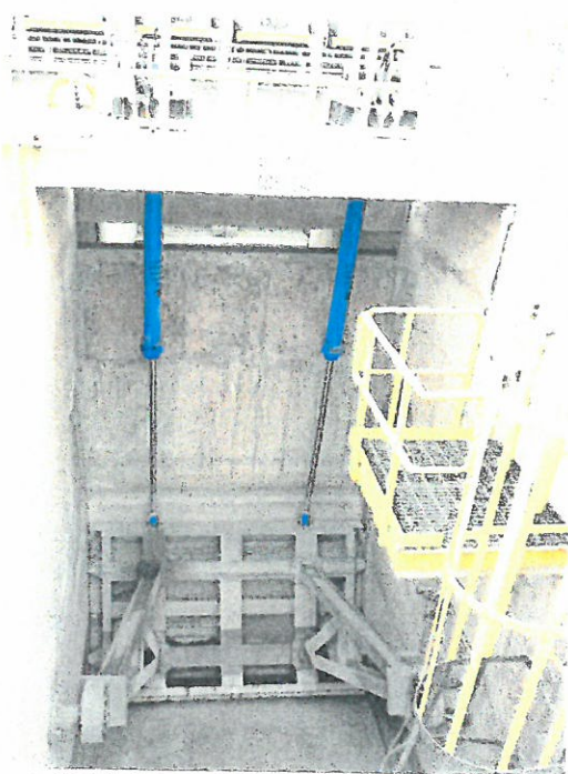
COMPUERTA RADIAL , BRAZOS DE IZAJE Y CILINDROS HIDRAULICOS
