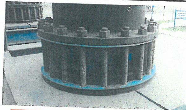
VALVULA CHECK EN LINEA DE IMPULSION
